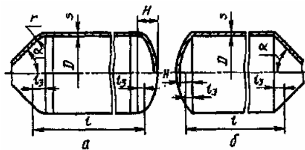
а - обечайка с отбортованными днищами, б - обечайка с неотбортованными днищами Черт. 2
