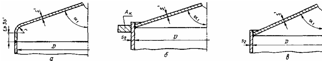
а - днище с тороидальным переходом, б - днище с укрепляющим кольцом, в - днище без тороидального перехода и укрепляющего кольца
